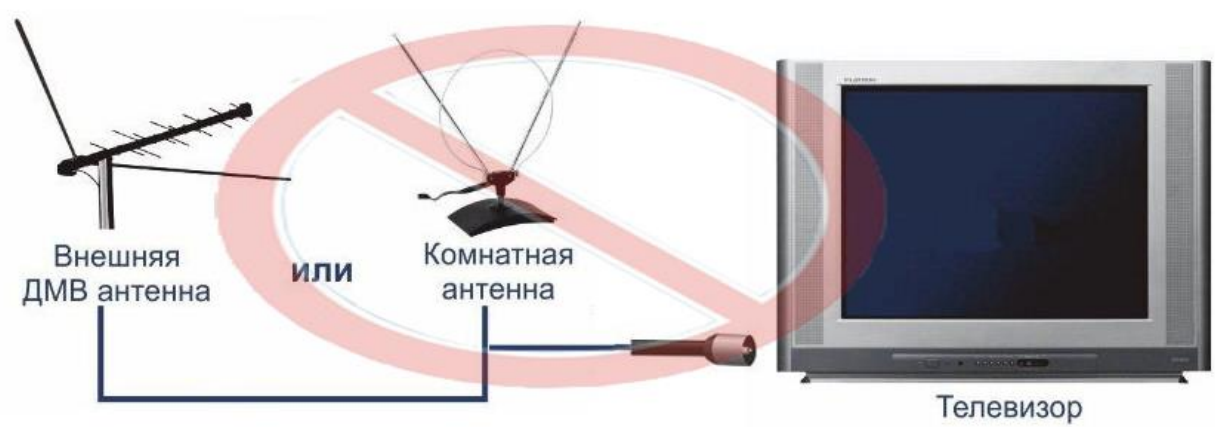
Фото 4. Схема приема аналогового телевизионного сигнала
